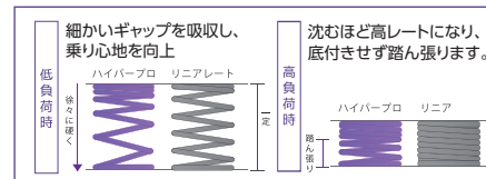
ストリートボックス(ツイン) フロントスプリング+リアショック
