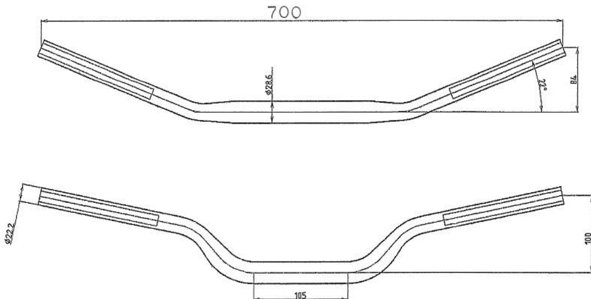
汎用テーパードハンドルバー寸法
