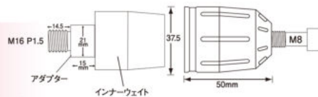
【重量320g/pc.】
