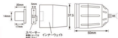
【重量338g/pc.】
